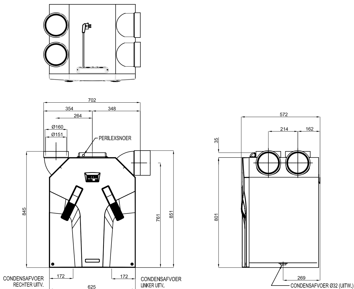
Afbeelding 0.1: Maatschets WHR 930
